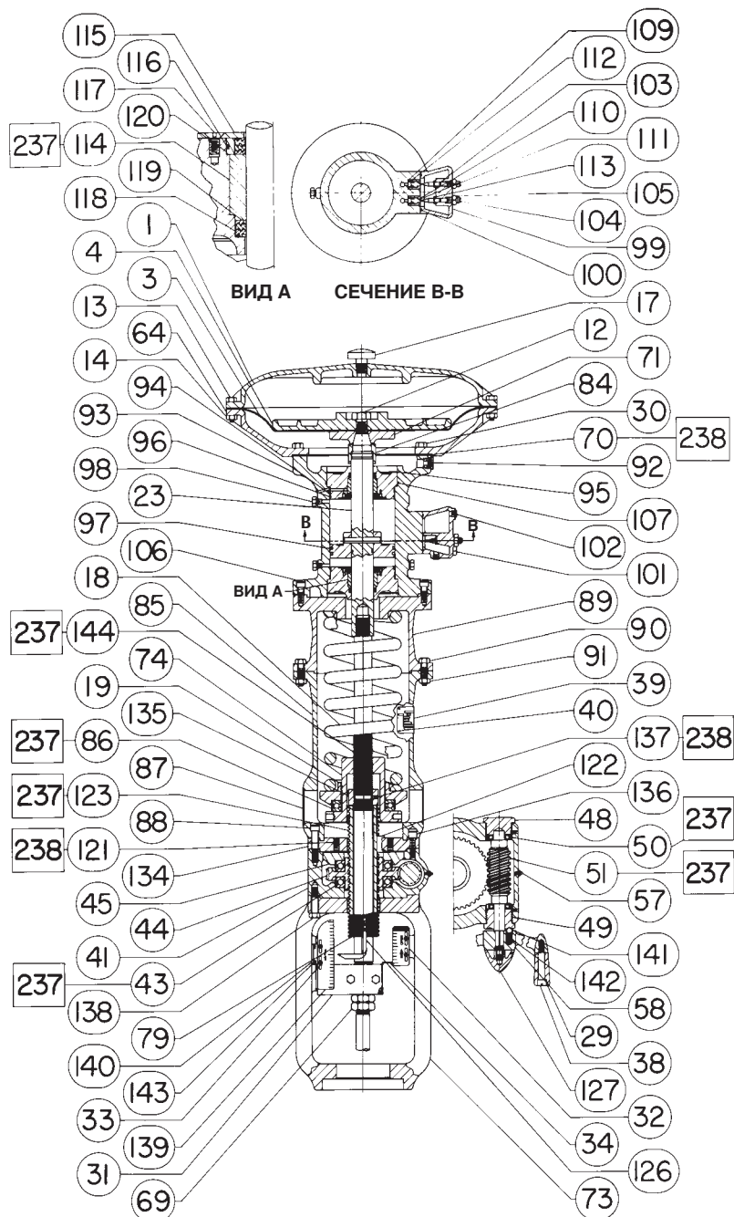
Рис. 8. Привод Fisher 667 размера 80 с ручным дублером бокового монтажа и гидравлическим демпфером
