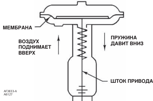
МЕМБРАНЫЙ ПРИВОД МОДЕЛИ 667 ОБРАТНОГО ДЕЙСТВИЯ
