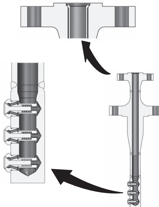
Рис. 3. Устройство пароохладителя DMA/AF-HTC компании Fisher
