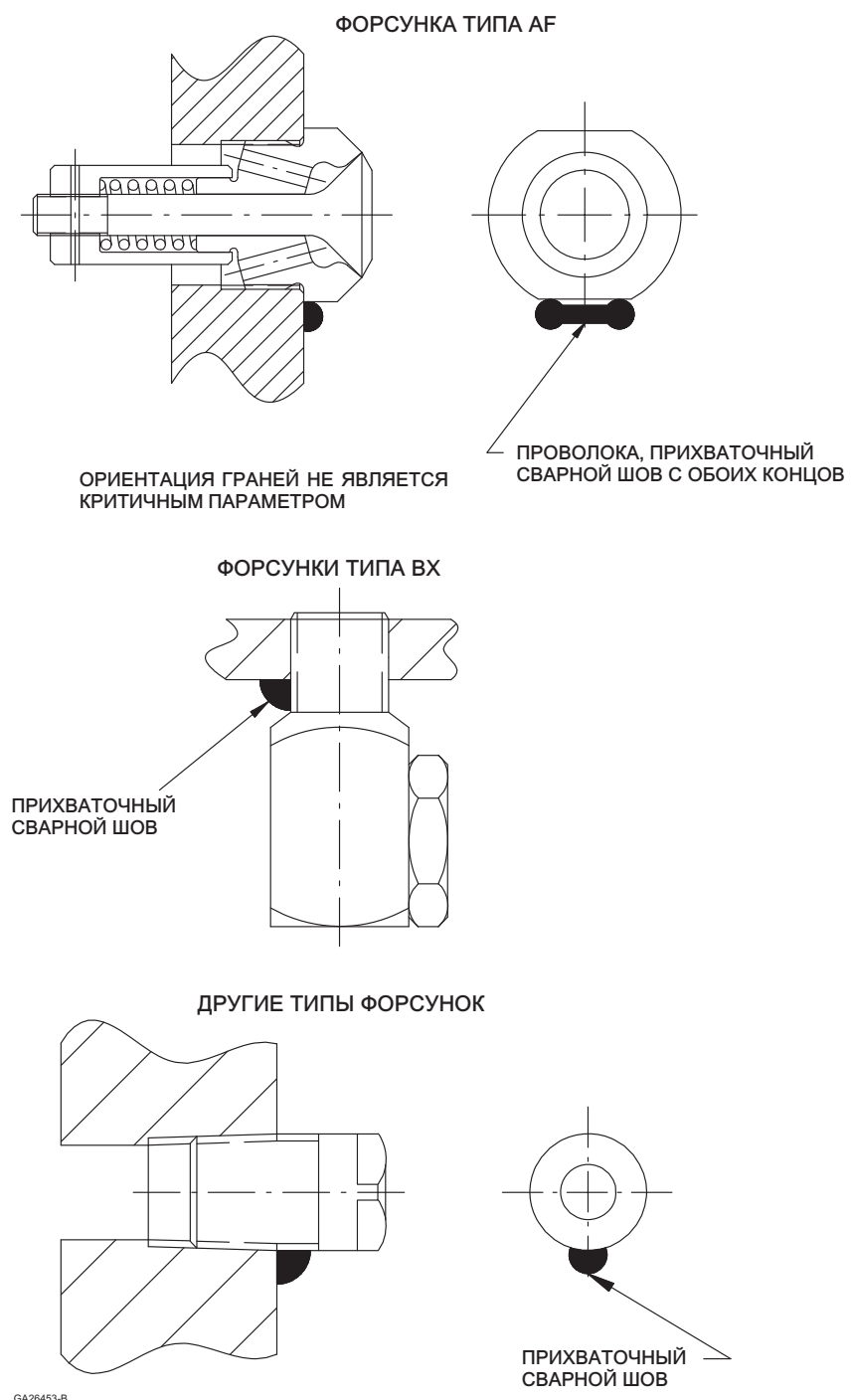
Рис. 8. Места прихваточных сварных швов распылительной форсунки
