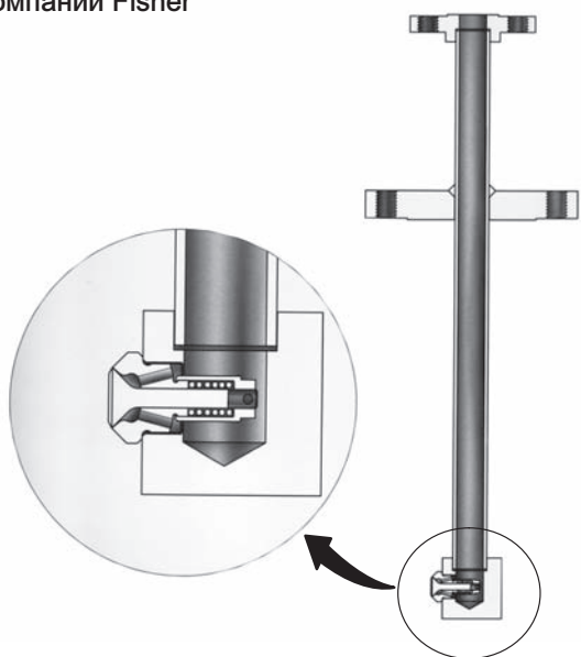
Рис. 2. Устройство пароохладителя DMA/AF компании Fisher
